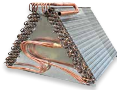
5mm A-frame (Marco en Forma A) Construido para HVAC Confort
